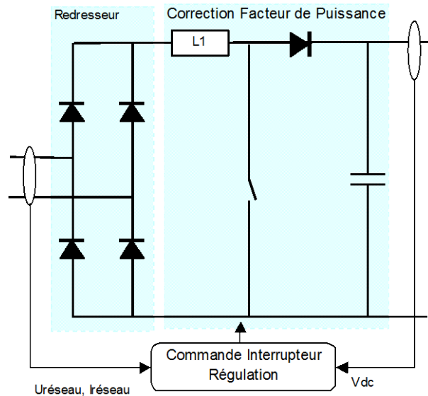
Etage d'entrée d'un variateur de vitesse avec correction du facteur de puissance
